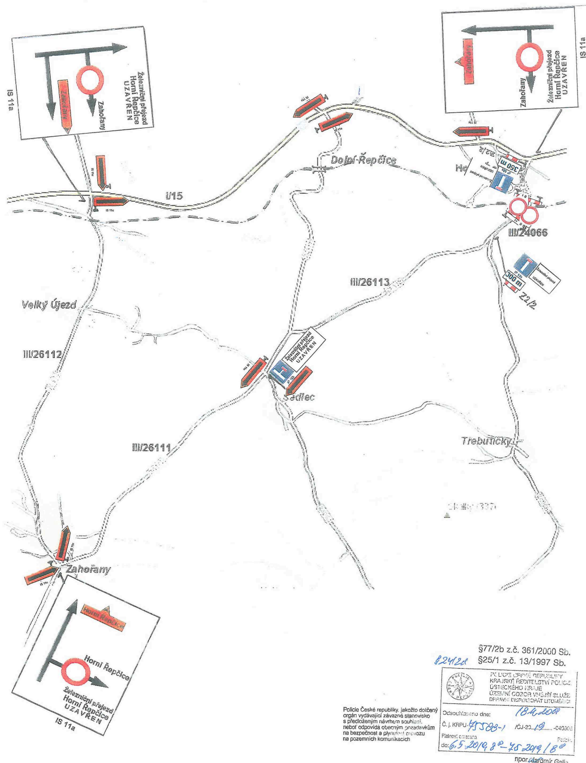
Návrh dopravního značení pro uzavírku komunikace III/ 24066 Horní Řepčice, v místě železničního přejezdu s tratí Lovosice – Česká Lípa, km 54,358
